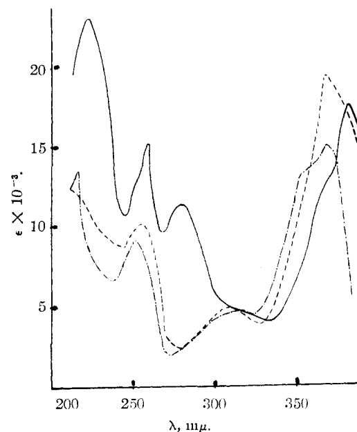
Fig. 3.—Ultraviolet light absorption of 3-cyano-6,7-benzo-2H-pyrido[1,2-a]pyrimidine (—), 3-acetyl-4-keto-4H-pyrido[1,2-a]pyrimidine (---), 3-cyano-4-keto-4H-pyrido[1,2-a]pyrimidine (-.-).
